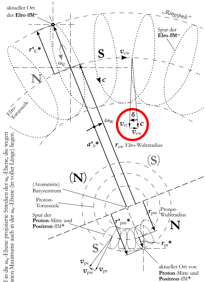
Bild 2 Schematischer Schrägblick auf die \omega_w -Ebene eines H-Atoms im Grundzustand – „von rechts unten“ keineswegs maßstäblich
